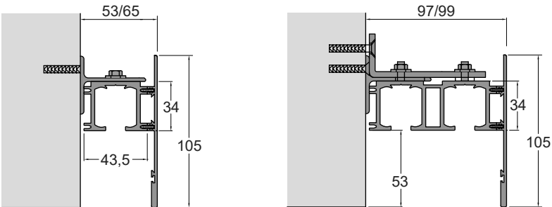
Binario ancorato a parete con mantovana in legno _Wall fixing track with wood valance
