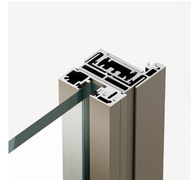
Sezione del profilo fermavetro 54 mm abbinato a stipite Cube per porte a battente o a bilico
