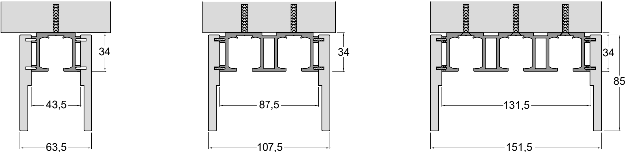
Binario ancorato a soffitto con mantovana in legno _Ceiling fixing track with wood valance
